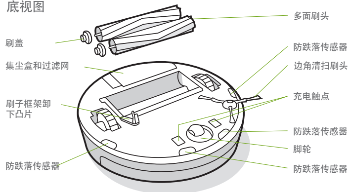
底视图
